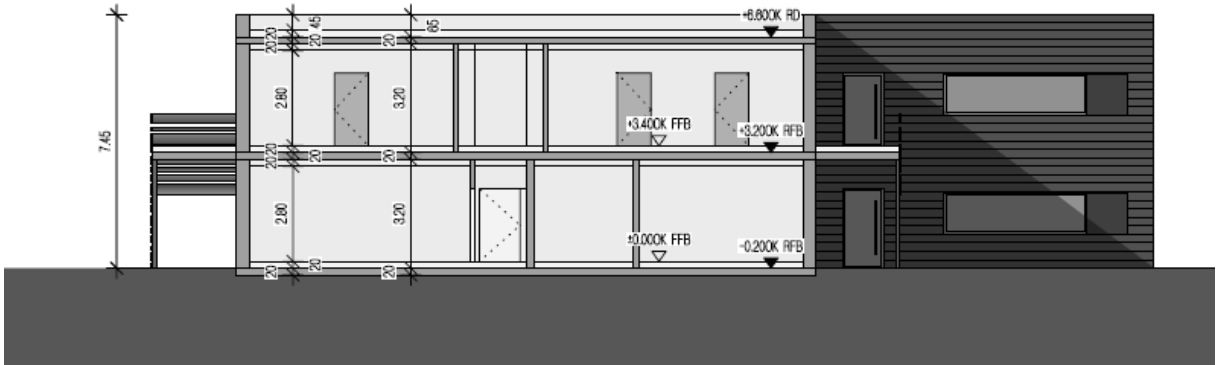
SCHNITT B-B
