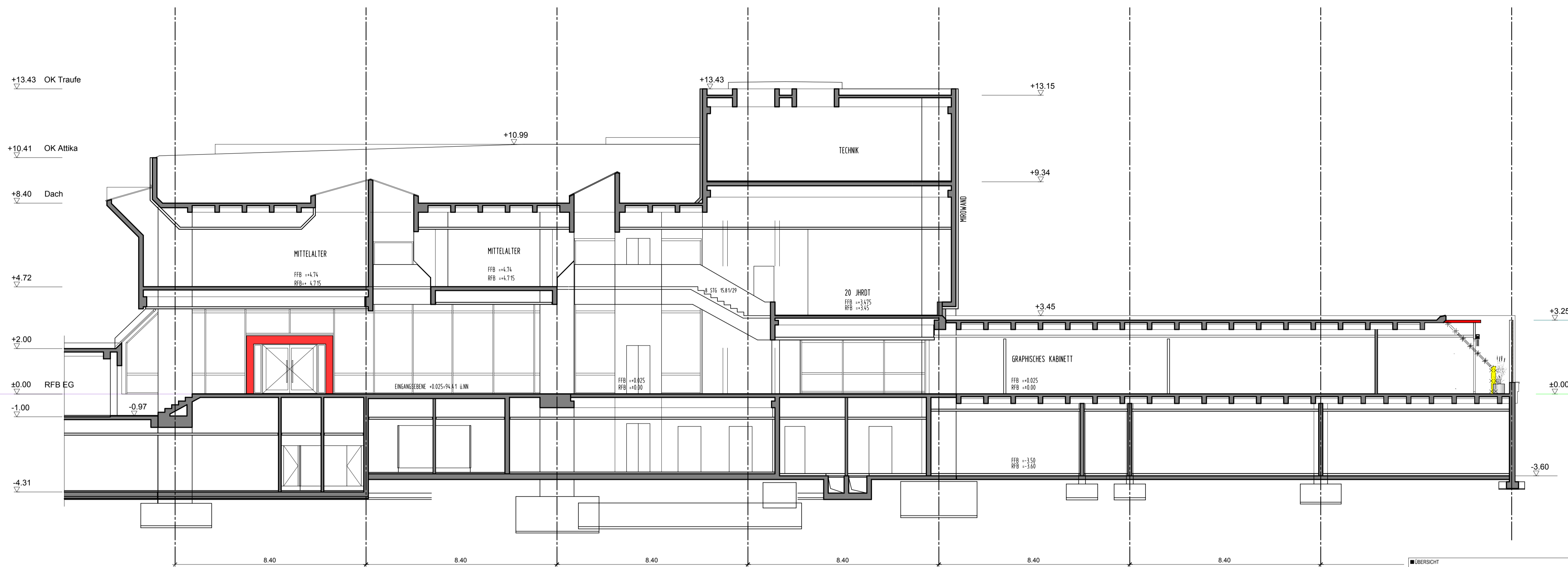
Schnitt A-A
