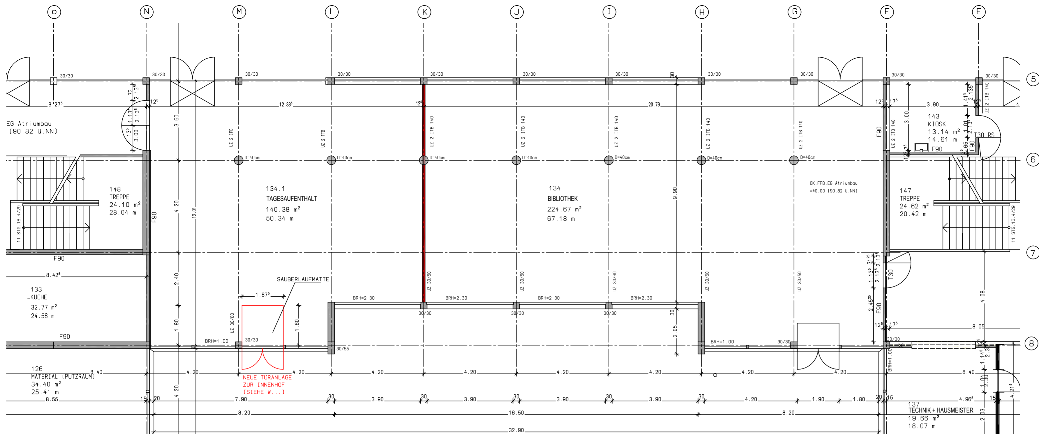
GRUNDRISS EG - AUSSCHNITT M: 1:100
