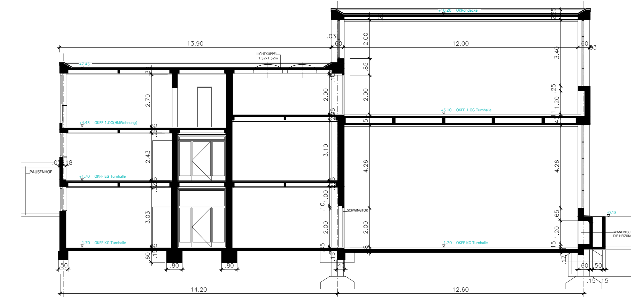
Schnitt C Turnhalle
