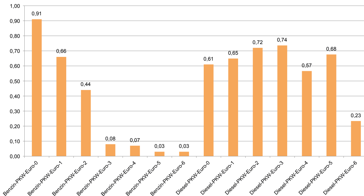
Abb. 16 Mittlere Emissionsfaktoren innerorts für Stickstoffoxide für Benzin- und Diesel-PKW in g/km, Bezugsjahr 2015 (Quelle: HBEFA 3.2)
